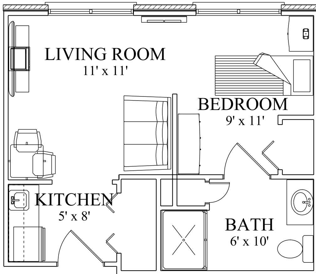
FLOORPLAN A SCALE: 340 SQ FT
